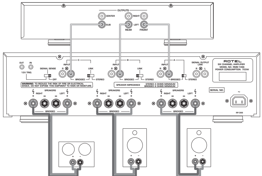
Figure 3: Bridged Connections Branchements en mode ponté (bridgé) Anschlußdiagramm bei Brückenschaltung Collegamenti a ponte Conexiones para Funcionamiento en Modo Puenteadado
