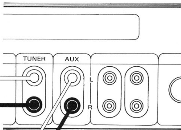
アンプのリアパネル AMPLIFIER (REAR PANEL)
