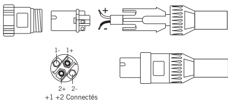
Câblage de passerelle
