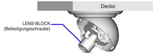
Deckenmontage (Standardposition)
