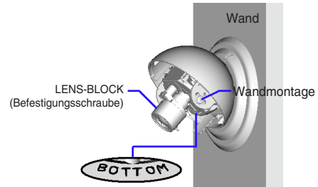
OBJEKTIV
