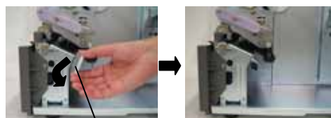
Slide guide
