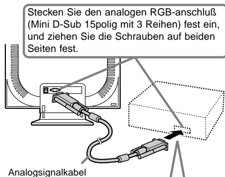
Analogsignalkabel
