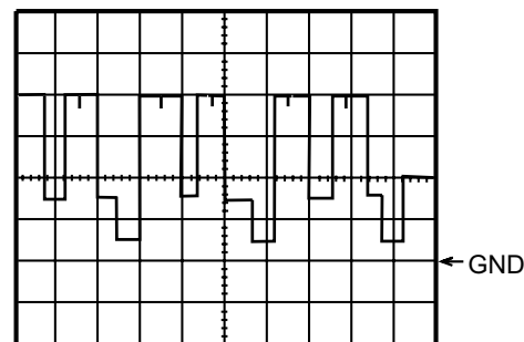
WF3 1DIV: 2V 20μsec Q 1511 Base
