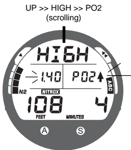
Fig. 65 - High PO2 Alarm Main
