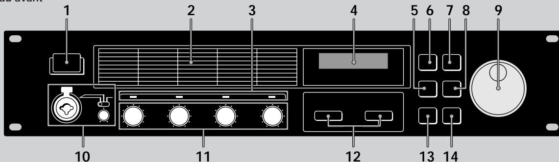
Panneau avant
