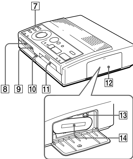
Compartiment à cassette
