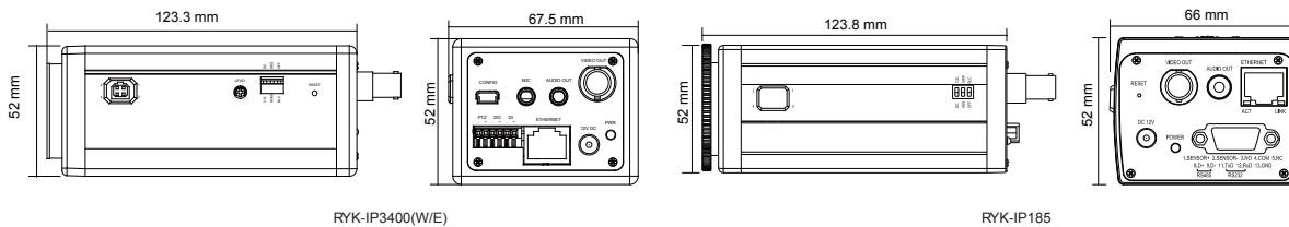
RYK-IP3400(W/E)
