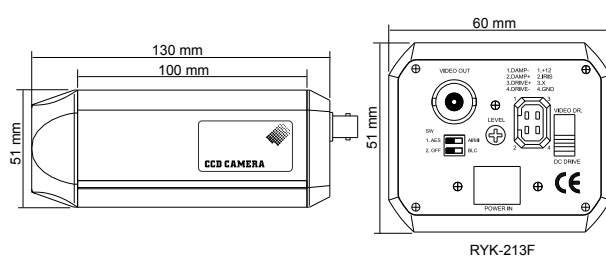
RYK-213F
