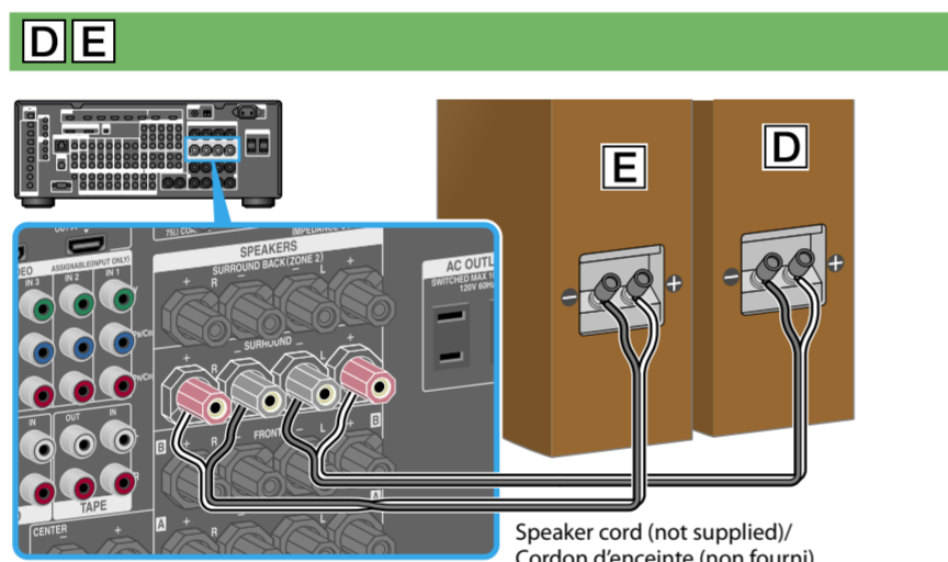
Speaker cord (not supplied)/ Cordon d'enceinte (non fourni)
