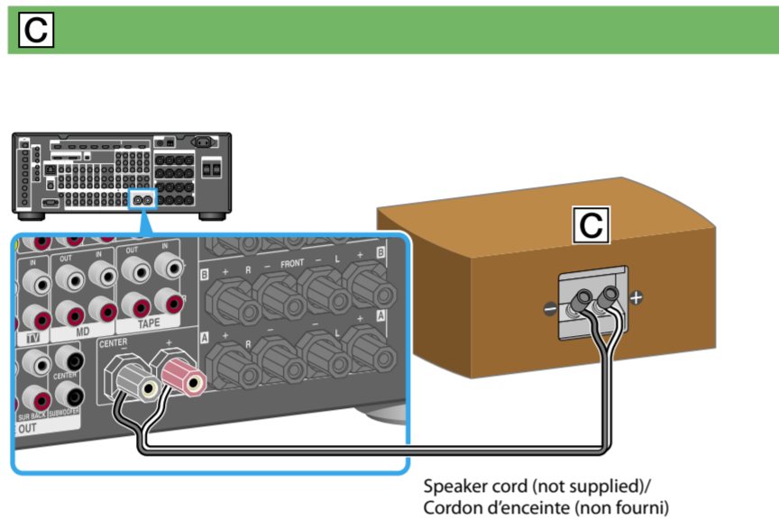
Speaker cord (not supplied)/ Cordon d'enceinte (non fourni)
