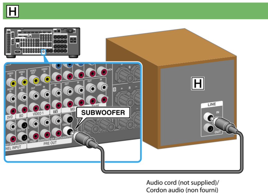
Speaker cord (not supplied)/ Cordon d'enceinte (non fourni)
