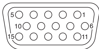
■ A-2 Sun XVR-100 繪圖加速器 HD15 接頭
