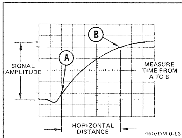
Fig. 19. Risetime.
