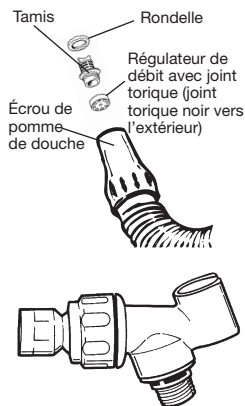
Régulateur de débit
