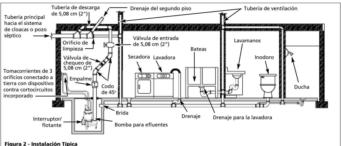
Figura 2 - Instalación Típica
