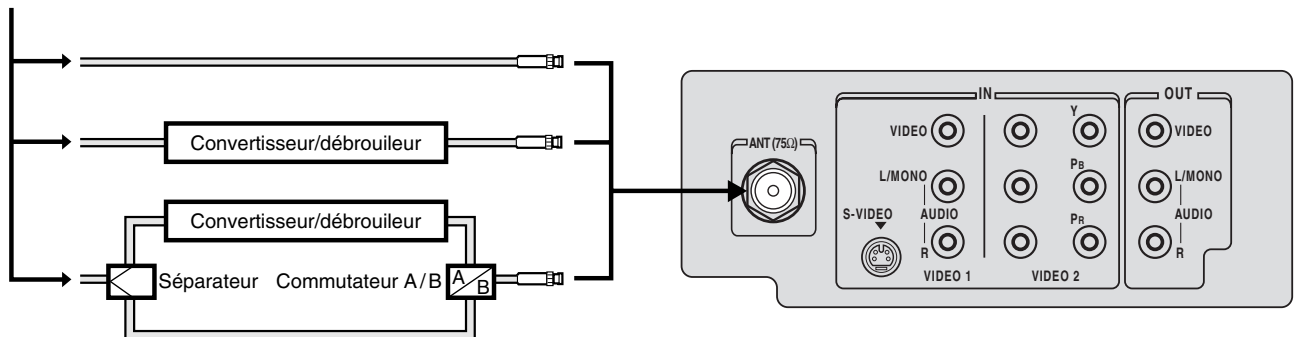
Câble du réseau de câblodistribution
