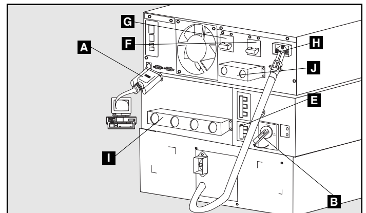
Модели 10 КВА (Задняя Панель)
