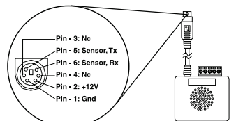
Рисунок 1: Разъем PS/2 датчика EnviroSense
