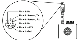
Figure 1 : Connecteur PS/2 EnviroSense
