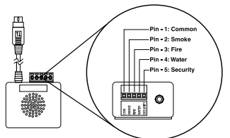
Рисунок 3: Подключение к EnviroSense устройств Contact Closure [замыкание контактов]
