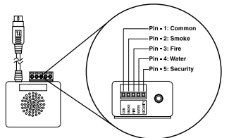
Figure 3 : Connexions Contact Closure [fermeture à contact] d'EnviroSense
