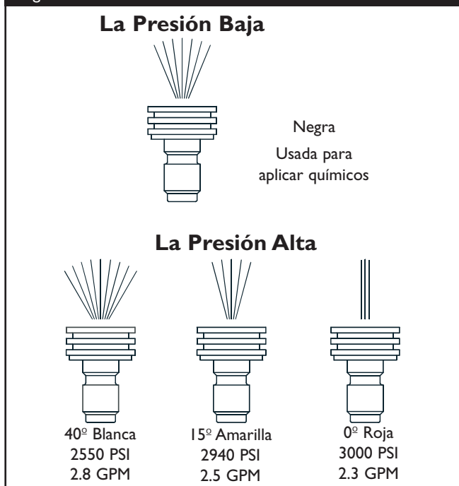
Figura 30 — Rocíe los Modelos del Roció de Punta
