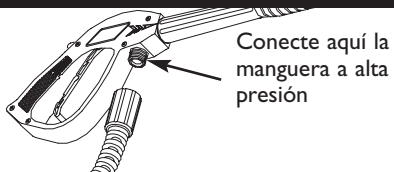
Figura 30 — Conecte la Manguera a alta Presión a la Pistola Rociadora
