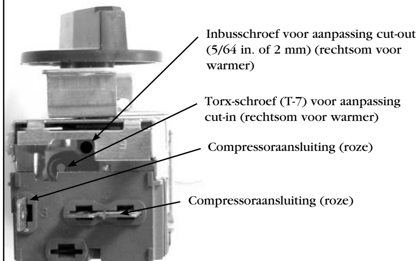
Danfoss thermostaat (alleen afstelling op grote hoogte!)
