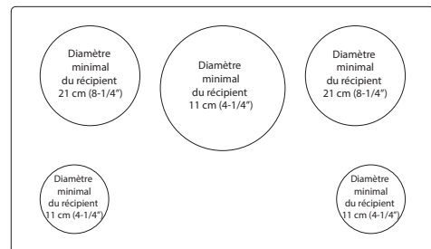
Fig 14b Table de cuisson d'une largeur de 91,4 cm (36"). Utilisez un récipient de la taille minimale indiquée pour chaque élément de cuisson.
