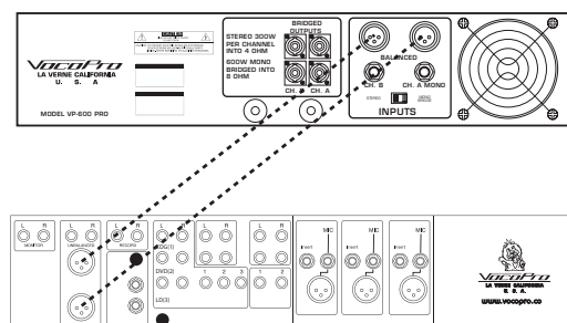
VP-600 PRO Amplifier
