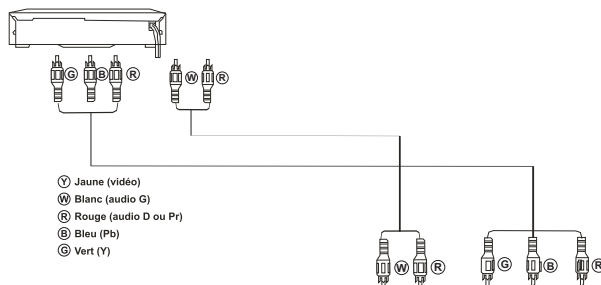
EQUIPEMENT VIDEO muni de connecteurs vidéo YPbPr
