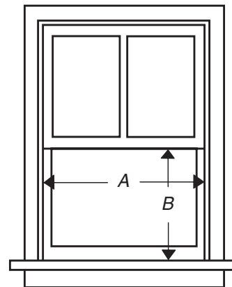
A. 28" (71,1 cm) mínimo a 40" (101,6 cm) máximo B. 16 1/4" (41,3 cm) mínimo
