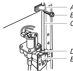
A. Bride du tube B. Vis de bride du tube C. Tube en plastique D. Écrou de compression E. Entrée du robinet
