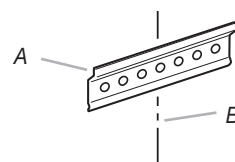
A. Bride de support inférieure B. Axe central tracé sur le mur
