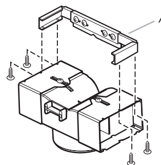
A. Bride de cache-conduit.
