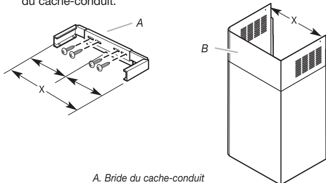
A. Bride du cache-conduit B. Section supérieure du cache-conduit
