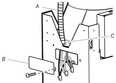
A. Conduit B. Couvercle de la boîte de connexion C. Connecteur de conduit
