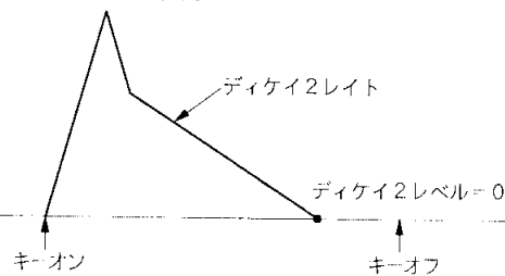
第31図 減衰音のエンベロープ例
