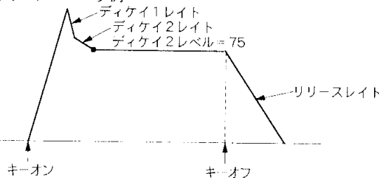
第32図 持続音のエンベロープ例
