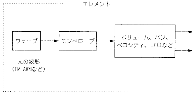
第9図 EOS B700エレメントの仕組み
