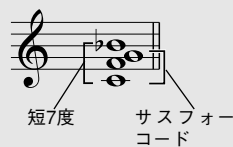
C7sus4
