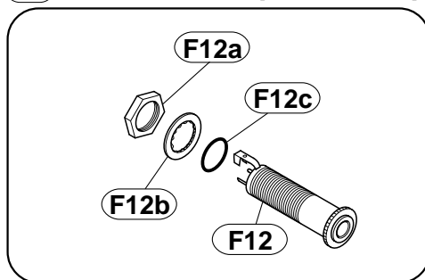
F12 Jack Installation (JACK 部詳細)
