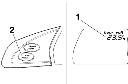
1 Hour meter/voltmeter
