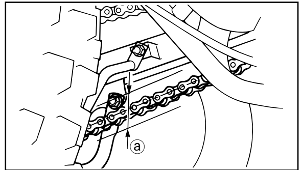
a. Drive chain slack
