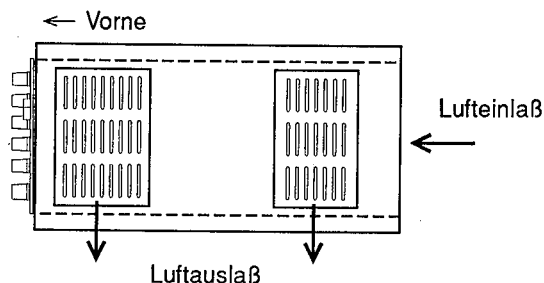
(Seitenansicht)
