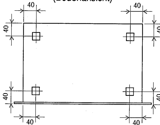
(Bodenansicht)
