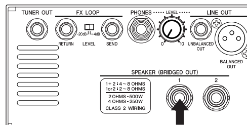
ヘッドアンプ/パワーアンプのスピーカー出力端子
