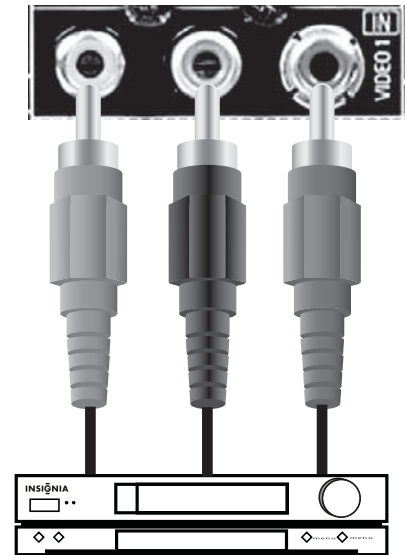
Conexión de video con calidad normal
