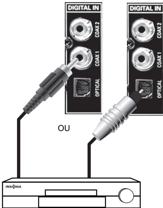
Connexion audio de qualité optimale
