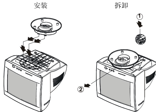
图一 底盘安装
