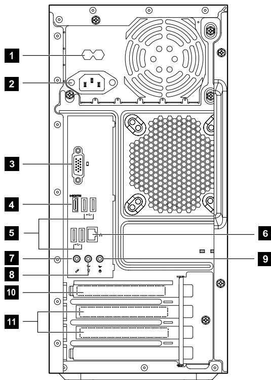
Lenovo H415
