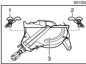
Fig. B: Al ángulo derecha de los ingletes 45°
