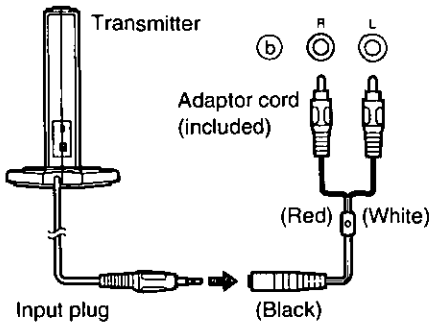
Input plug
