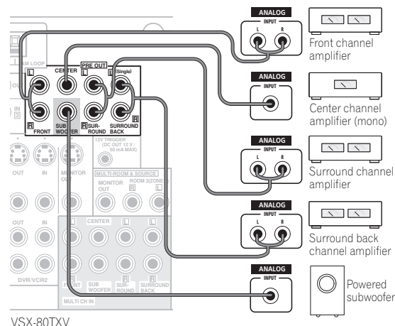
VSX-80TXV
