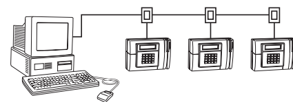
RS485 LAN Configuration
