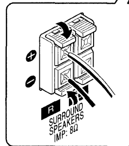
Enceintes surround
