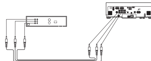
Komponent-Kabel anschließen Videokabel anschließen
