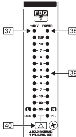
Fig. 2.16: Level meter
