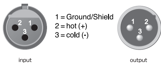
図 5.1 : XLR 接続
