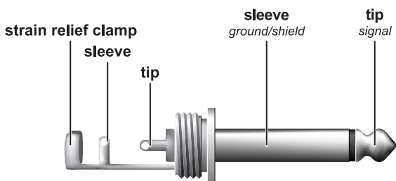
図 5.2 : 6.3 mm モノラルフォンプラグ
