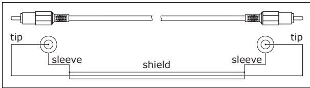
Fig. 4.5: RCA cable
