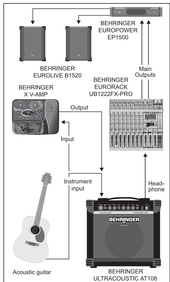
Fig. 2.2: Live setup
