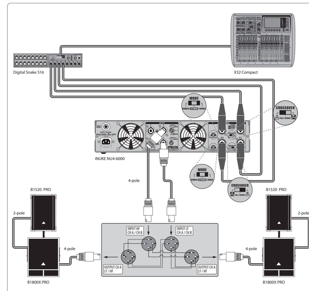
Horizontal Bi-amping/Bi-amplificación horizontal/Bi-amplification horizontale/Horizontal Bi-Amping/Bi-amplificação Horizontal
