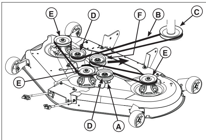
Figura 18. Encaminamiento de la correa del cortacésped
