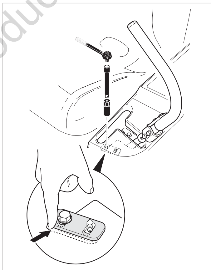
Figura 15. Ajuste de equilibrio de velocidad
