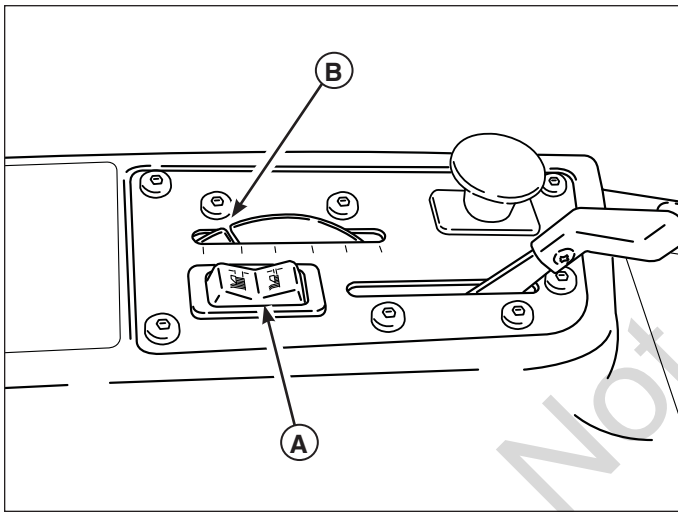
Figura 16. Ajuste de la altura de corte
